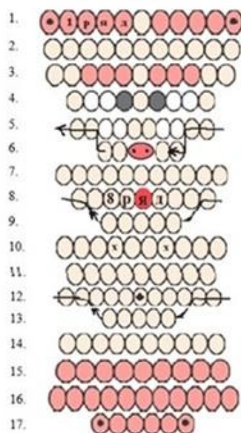
Общая схема плетения Рис.1
